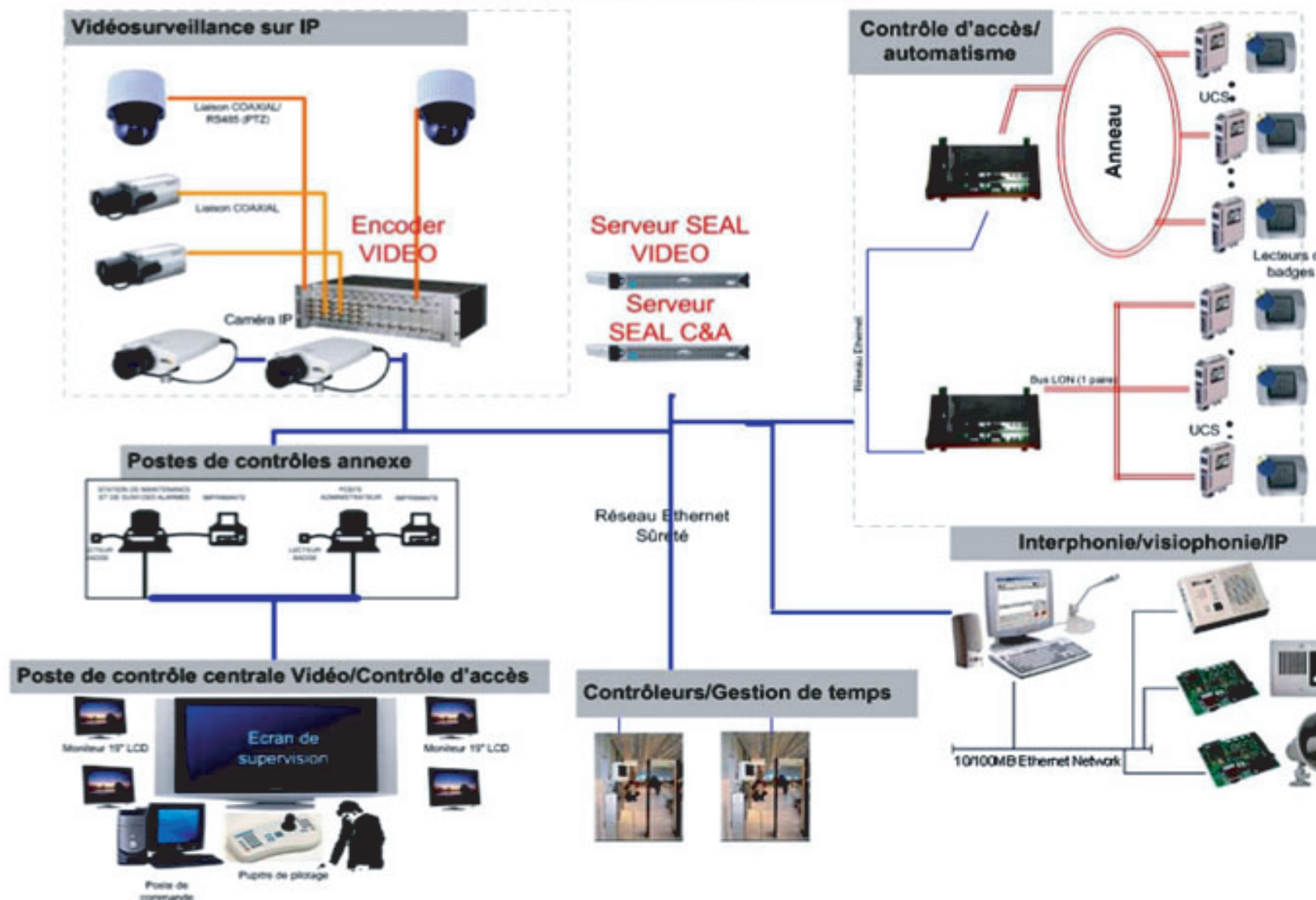
Schéma de principe des systèmes de sûreté SEAL
